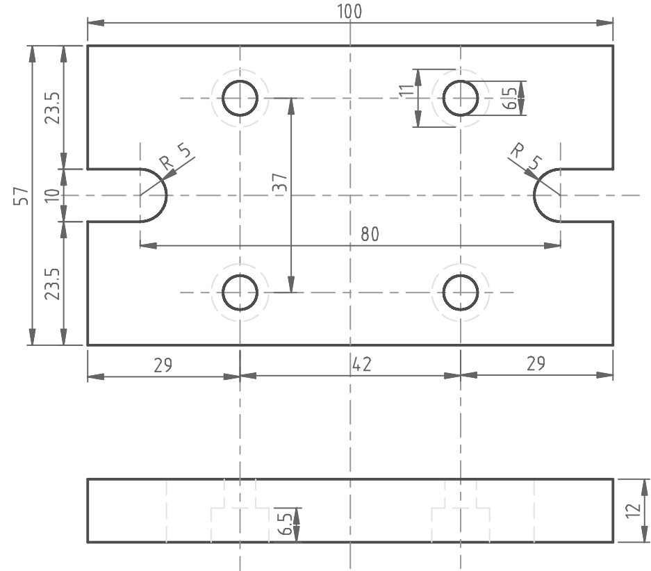
Bodemplaat / Base plate
