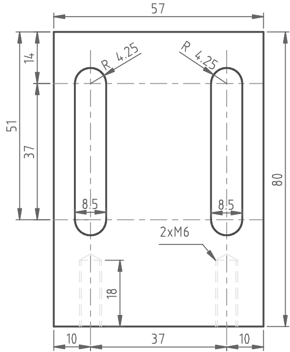
Zijflens / Column 2X
