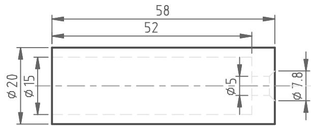
Kruk handvat Crank handle
