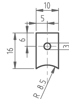
Bout geleider klem Bolt guide clamp
