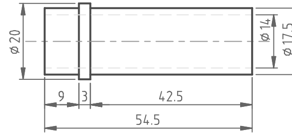
Boutgeleider Bolt guide
